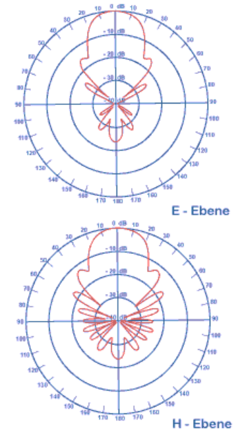
Richtdiagrammen
