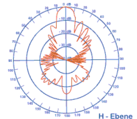
H - Ebene
