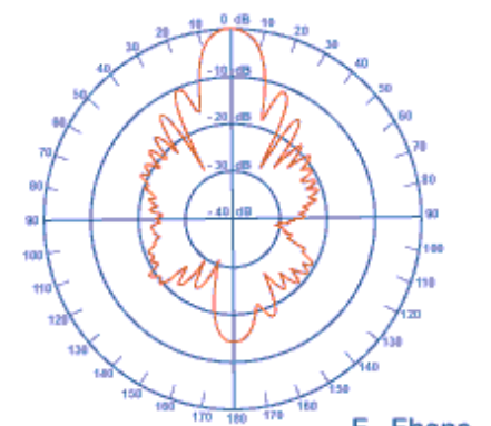
E - Ebene
